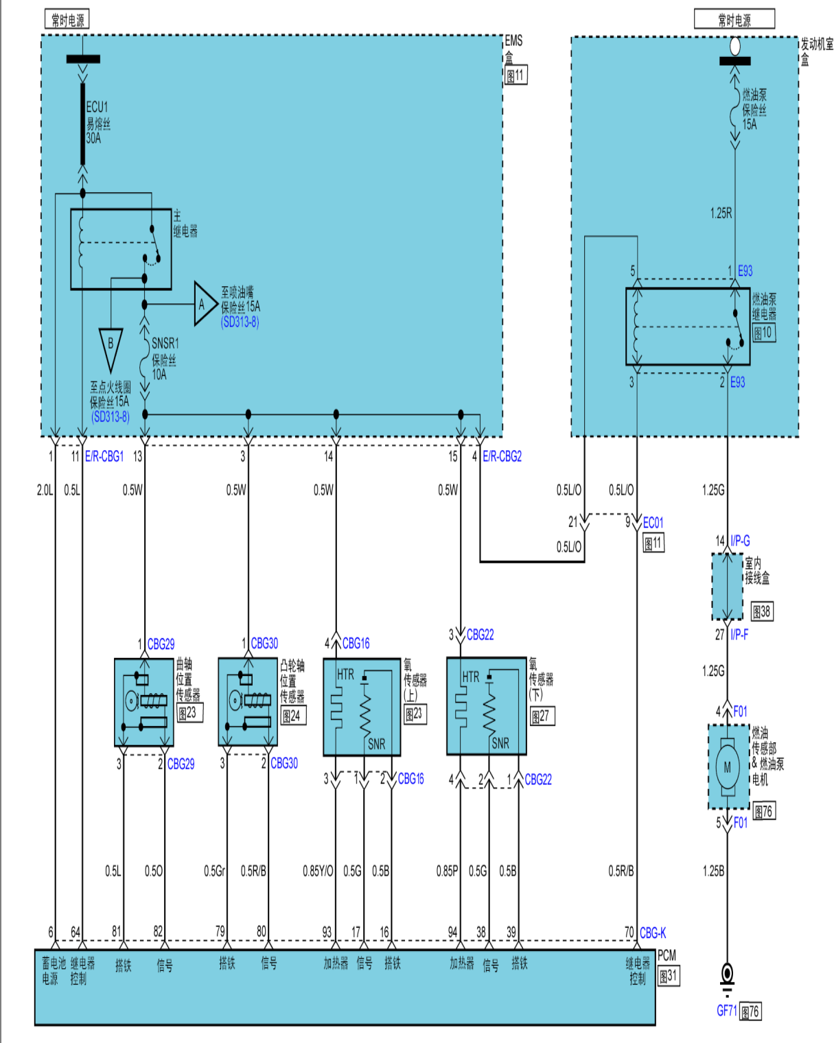
MFI 控制系统(G4GB) (1)
